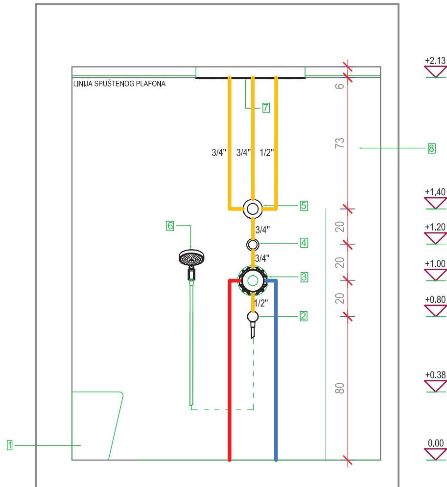
PRESEK A-A
