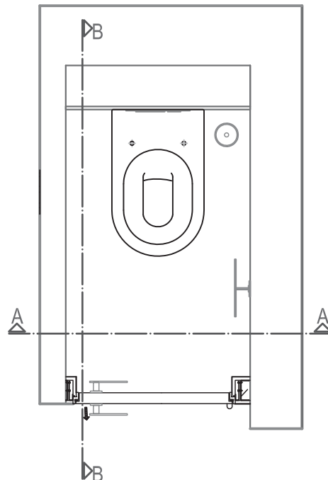
OSNOVA
