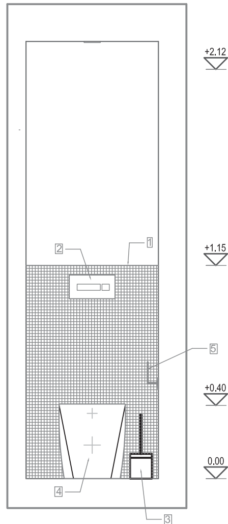
PRESEK A-A
